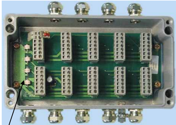
4 Stück Überspannungsableiter
